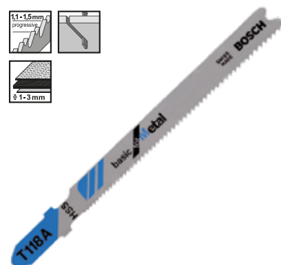
Segueta T118A caladora metal
