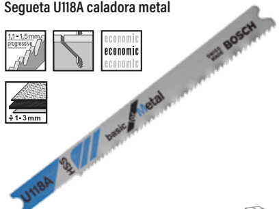
Segueta U118A caladora metal
